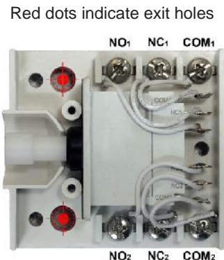
... Wiring ...
